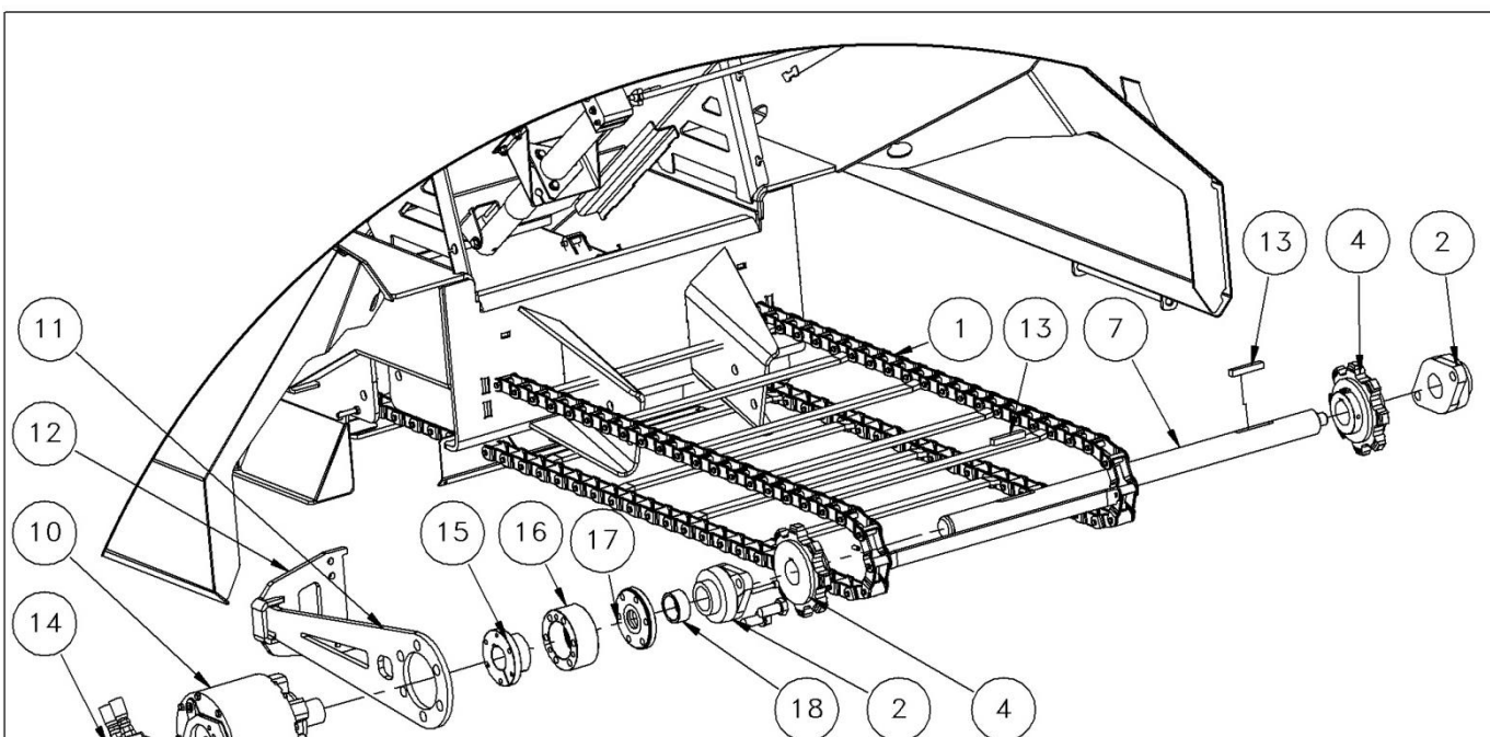
VUE AVANT DE LA CHAÎNE ET DU SYSTÈME MENANT CHAIN FRONT VIEW AND DRIVING SYSTEM
