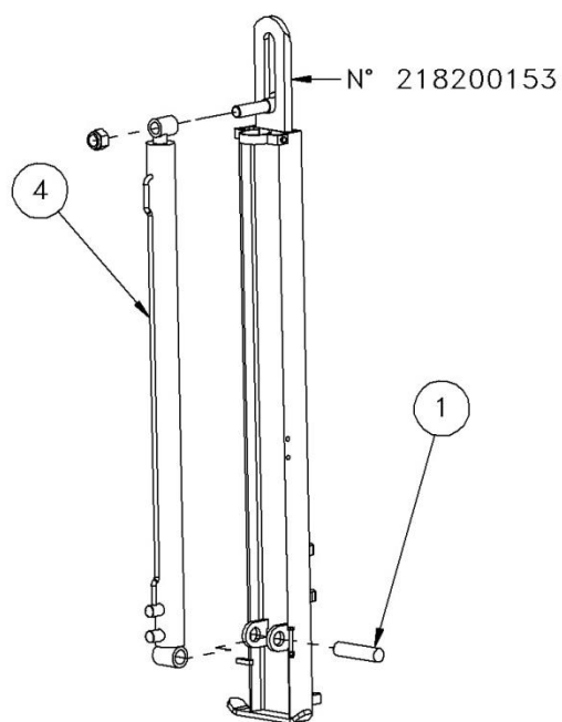
VUE C COLONNE AVANT HYDR. 48'' VIEW C 48'' HYDR. FRONT POST
