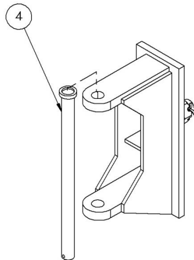
PENTURE FIXE/FIXE HINGE KIT N° 215220045
