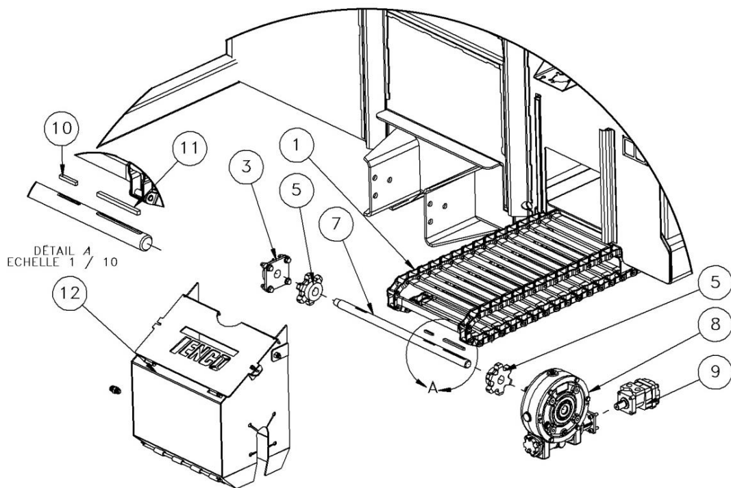
VUE AVANT DE LA CHAÎNE ET DU SYSTEME MENANT CHAIN FRONT VIEW AND DRIVING SYSTEM
