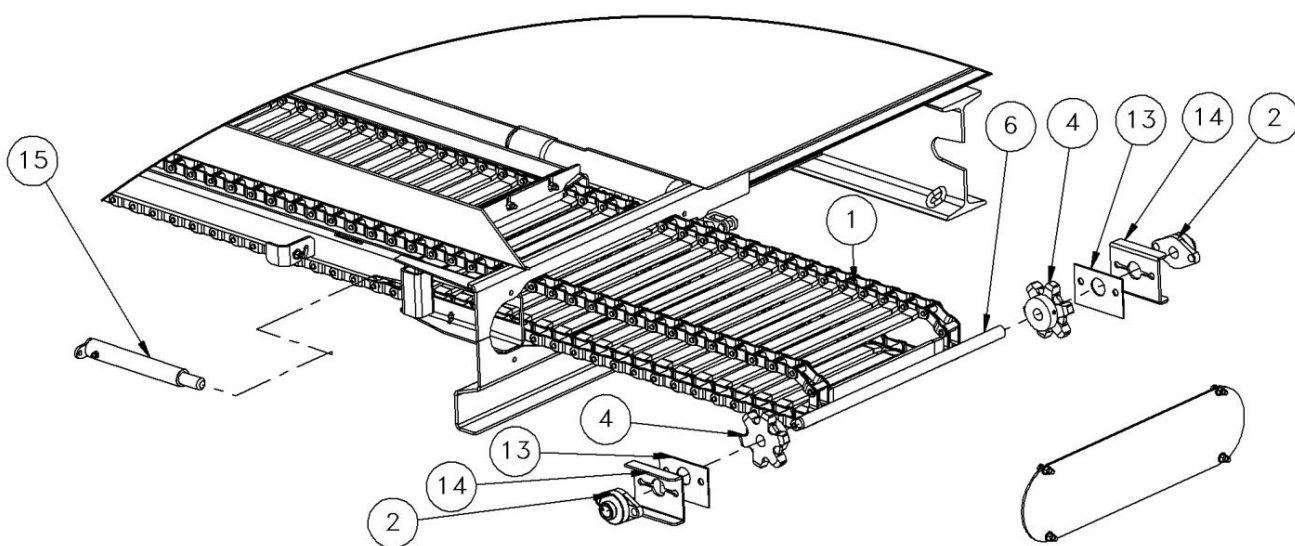
VUE ARRIERE DE LA CHAÎNE ET DE LA PORTE D'ACCÈS CHAIN REAR VIEW AND ACCESS DOOR
