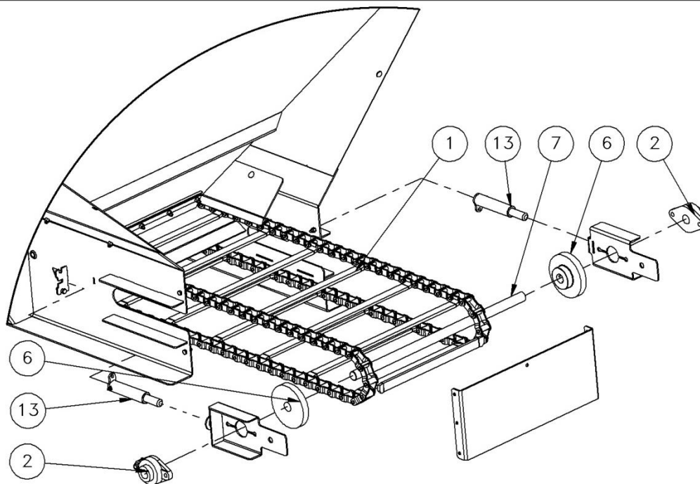
VUE AVANT DE LA CHAÎNE ET DE LA PORTE D'ACCÈS CHAIN FRONT VIEW AND ACCESS DOOR
