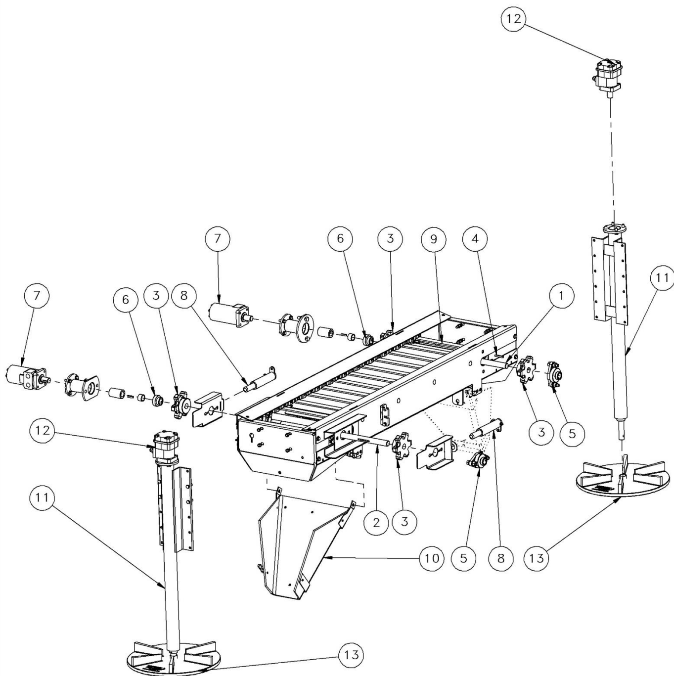
KIT PRÉSENTÉ N° 212300261 PRESENTED KIT N° 212300261
