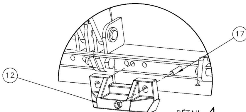
DÉTAIL A ECHELLE 1 / 8
