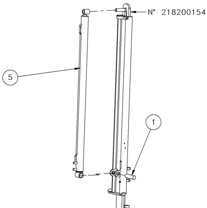
VUE D COLONNE AVANT HYDR. 60'' VIEW D 60'' HYDR. FRONT POST
