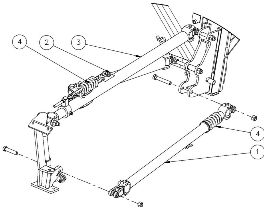
VUE ÉCLATÉE BRAS DE POUSSÉ 27'' EXPLODED VIEW 27'' PUSH ARM
