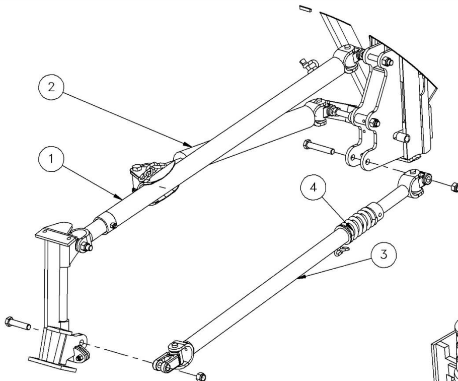
VUE ÉCLATÉE BRAS DE POUSSE 25'' EXPLODED VIEW 25'' PUSH ARM
