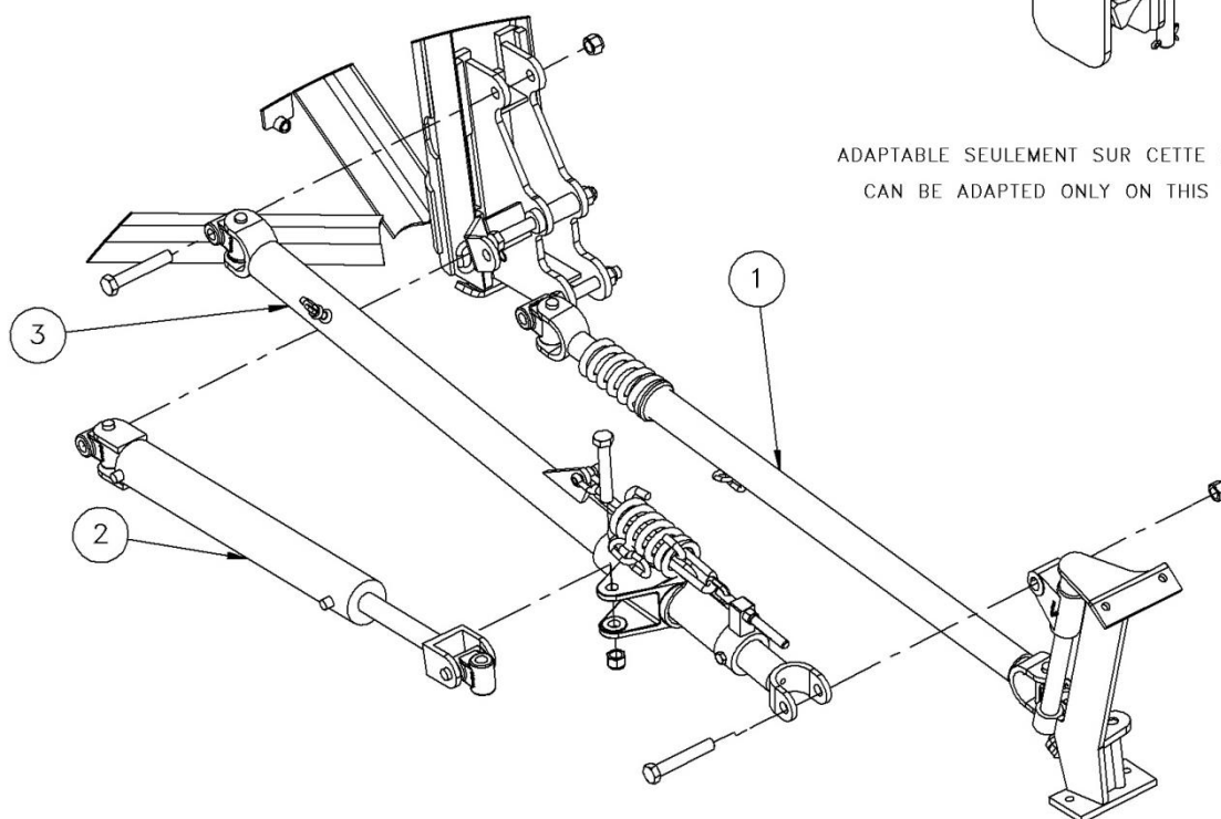
VUE ÉCLATÉE BRAS DE POUSSÉ 27'' EXPLODED VIEW 27'' PUSH ARM
