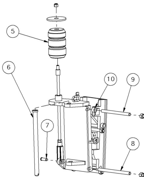
PENTURE 20 DEGRÉS/20 DEGREE HINGE KIT N° 215220047
