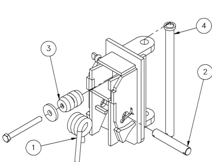
PENTURE 20 DEGRÉS/20 DEGREE HINGE KIT N° 215220047
