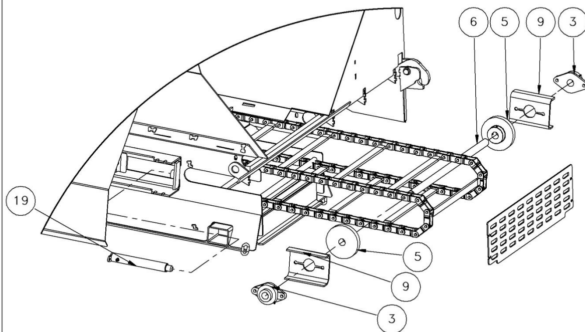
VUE ARRIERE DE LA CHAÎNE ET PORTE D'ACCÈS CHAIN REAR VIEW AND ACCESS DOOR
